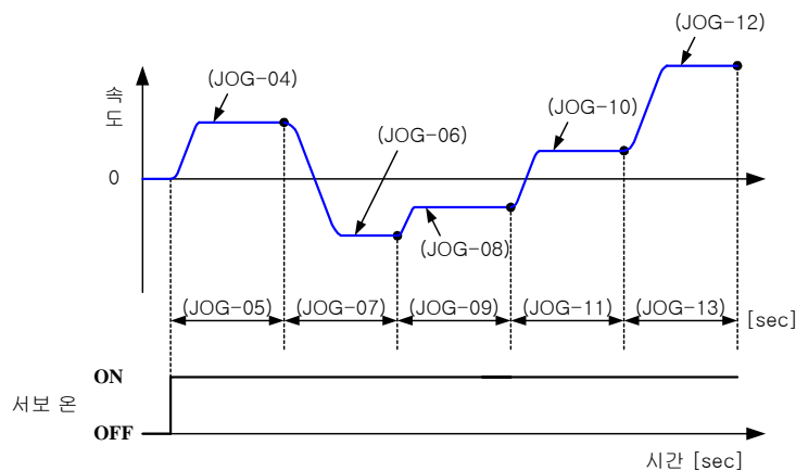
[오토 조그 모드 1(속도-시간)]
