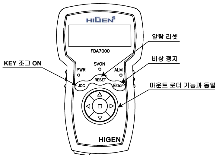
[ 디지털 로더의 개략도 ]
