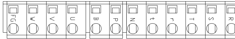
[ FDA7004/7004B ~ FDA7010 주회로 단자대 ]
